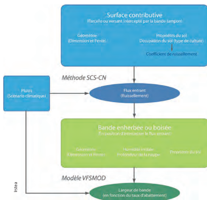
Figure 32 - Schéma de principe de la méthode de dimensionnement des bandes enherbées ou boisées pour l'atténuation des transferts de pesticides par ruissellement.
