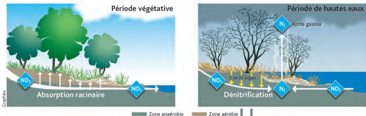
Figure 28 - Complémentarité des processus d'atténuation des transferts de nitrate d'une zone boisée de bas-fond selon la saison [d'après Maridet, 1995]
