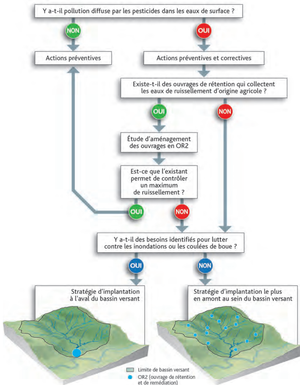
Figure 36 - Schéma de décision pour l'aménagement ou l'implantation d'ouvrage de rétention et de remédiation [d'après Regazzoni et al., 2011].
