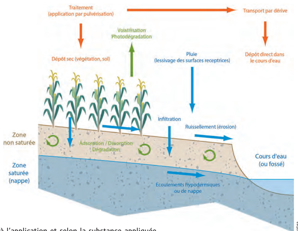
Fig. 22 - Processus de rétention, de dissipation et de dispersion des pesticides dans le milieu.
