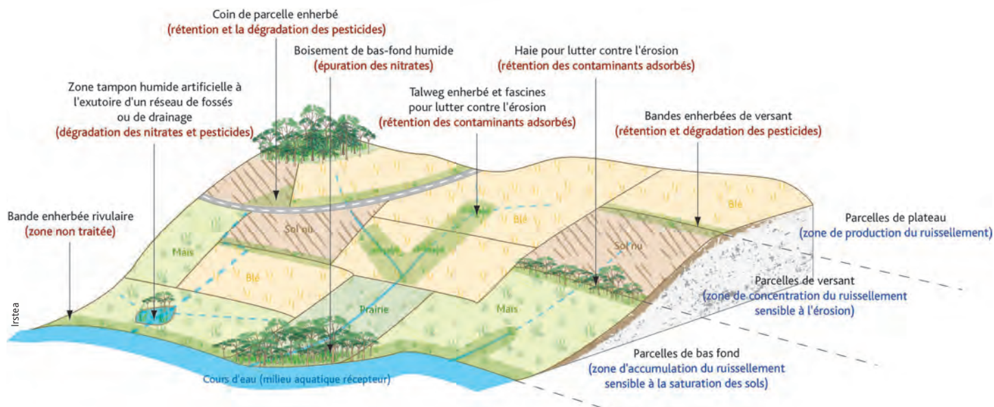
Fig.27 - Un exemple d'aménagement de zones tampons dans un versant à forte dominante agricole : une diversité de solutions peut être proposée pour répondre aux différentes problématiques rencontrées
