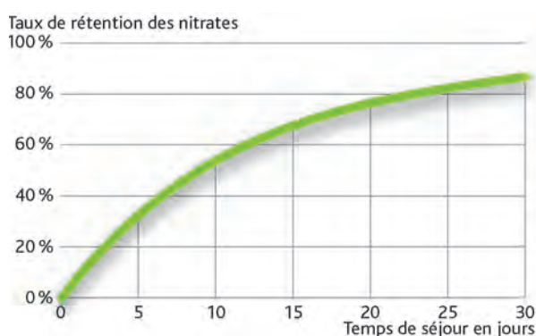
Figure 30 - Courbe des taux d'abattement des teneurs en nitrate (%) en fonction du temps de séjour dans une ZTHA, à température constante de 20°C [basée sur l'approche « tanks in series » de Kadlec et Wallace, 2008]
