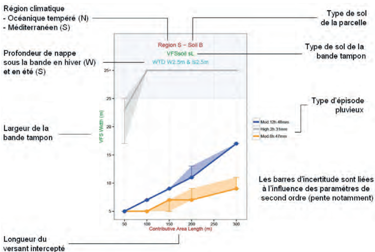
Figure 34 - Exemple de graphique de synthèse proposé par Irstea pour le dimensionnement des bandes tampons végétalisées dans un but d'atténuation des transferts de pesticides par ruissellement. Le détail des différents paramètres pris en compte est présenté dans Carlier et Lauvernet (2014).
