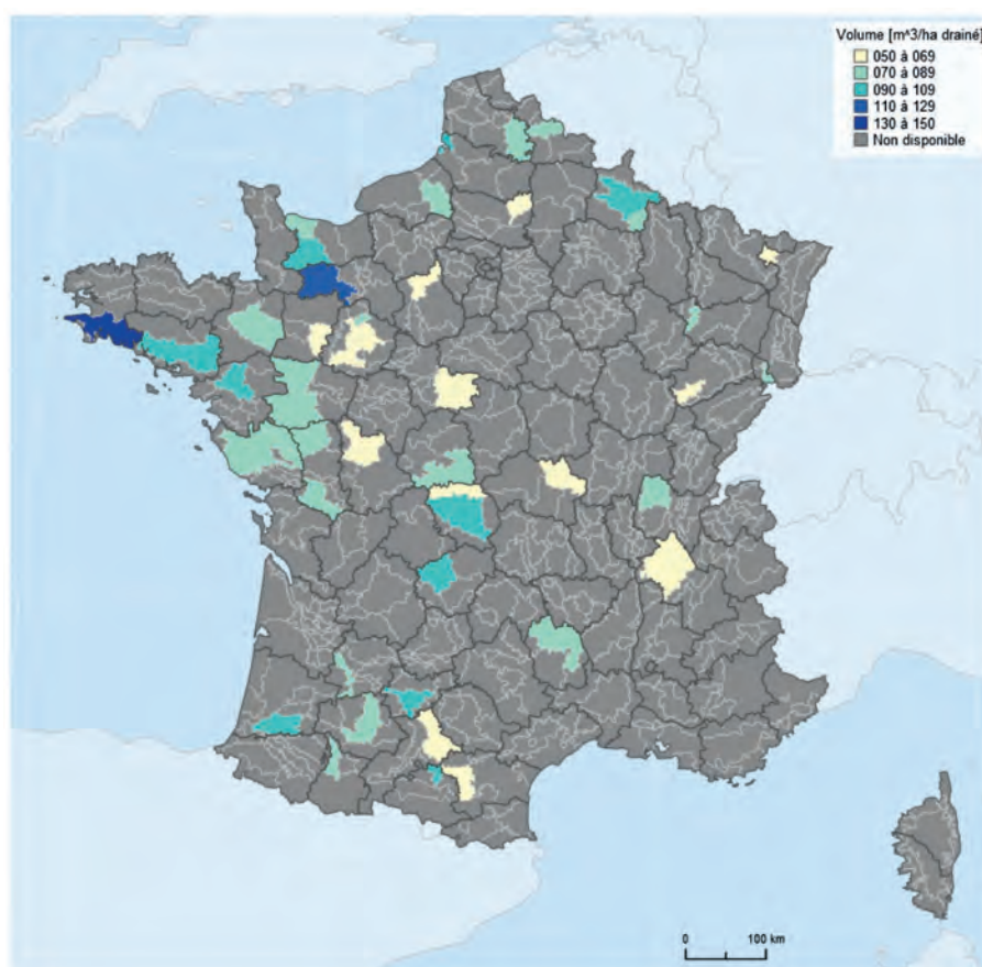
Figure 29 - Volumes des zones tampons humides artificielles (en m 3 par hectare drainé) préconisées par Tournebize et al. (2015) pour l'épuration du nitrate par petites régions agricoles
