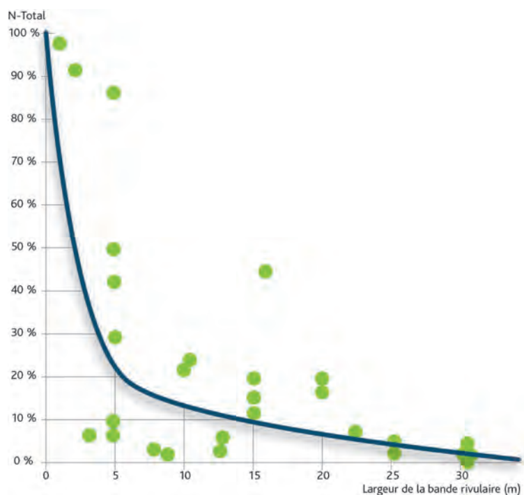
Figure 31 - Taux d'abattement attendu des teneurs en azote total (azote minéral et organique) en fonction de la largeur de la ripisylve [d'après Maridet, 1995]
