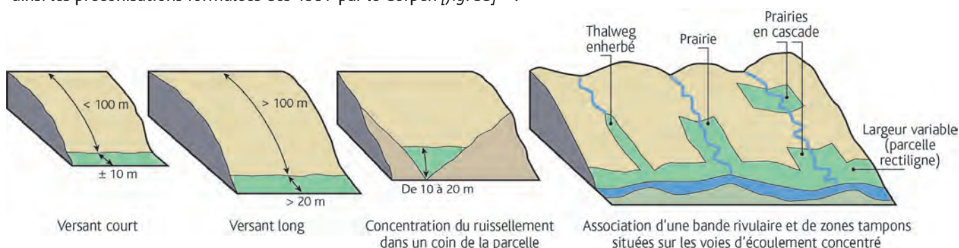
Figure 33 - Préconisations formulées par le Corpen en matière de largeur et de géométrie des bandes tampons végétalisées pour l'atténuation des transferts de produits phytosanitaires par ruissellement [d'après Corpen, 1997].
